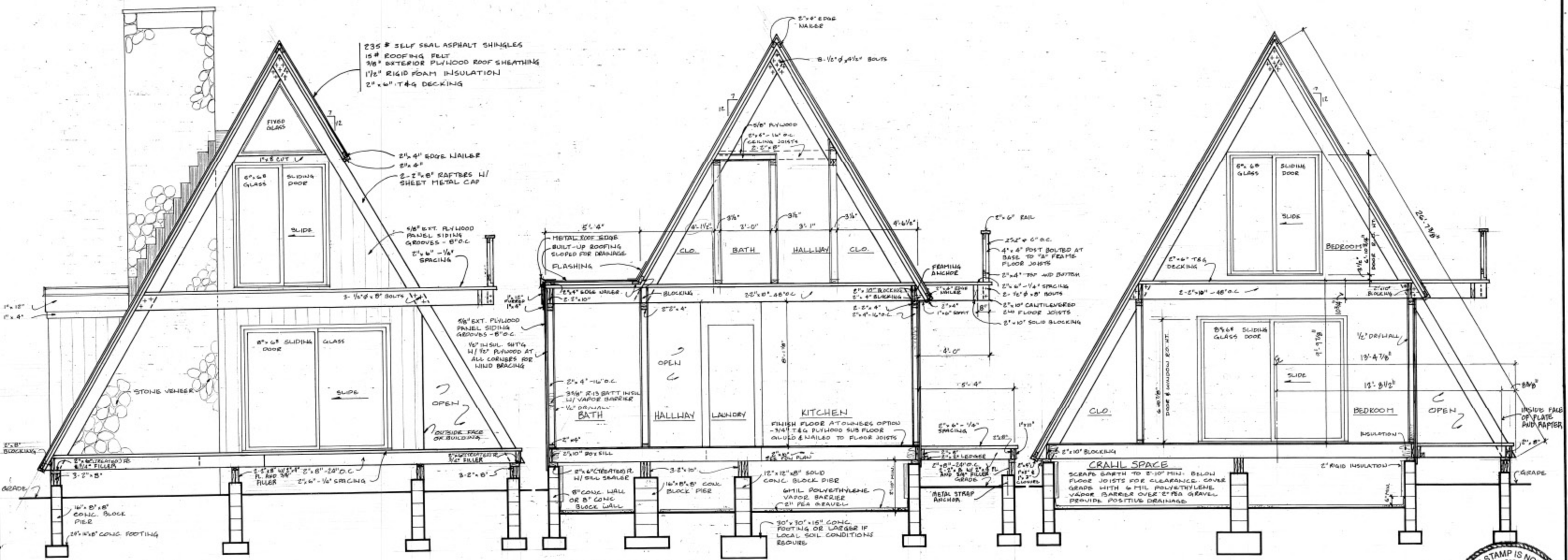
SECTION "C 5" SCALE: 3/8" = 1'-0"
