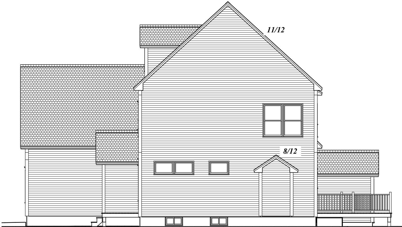
Right Elevation
