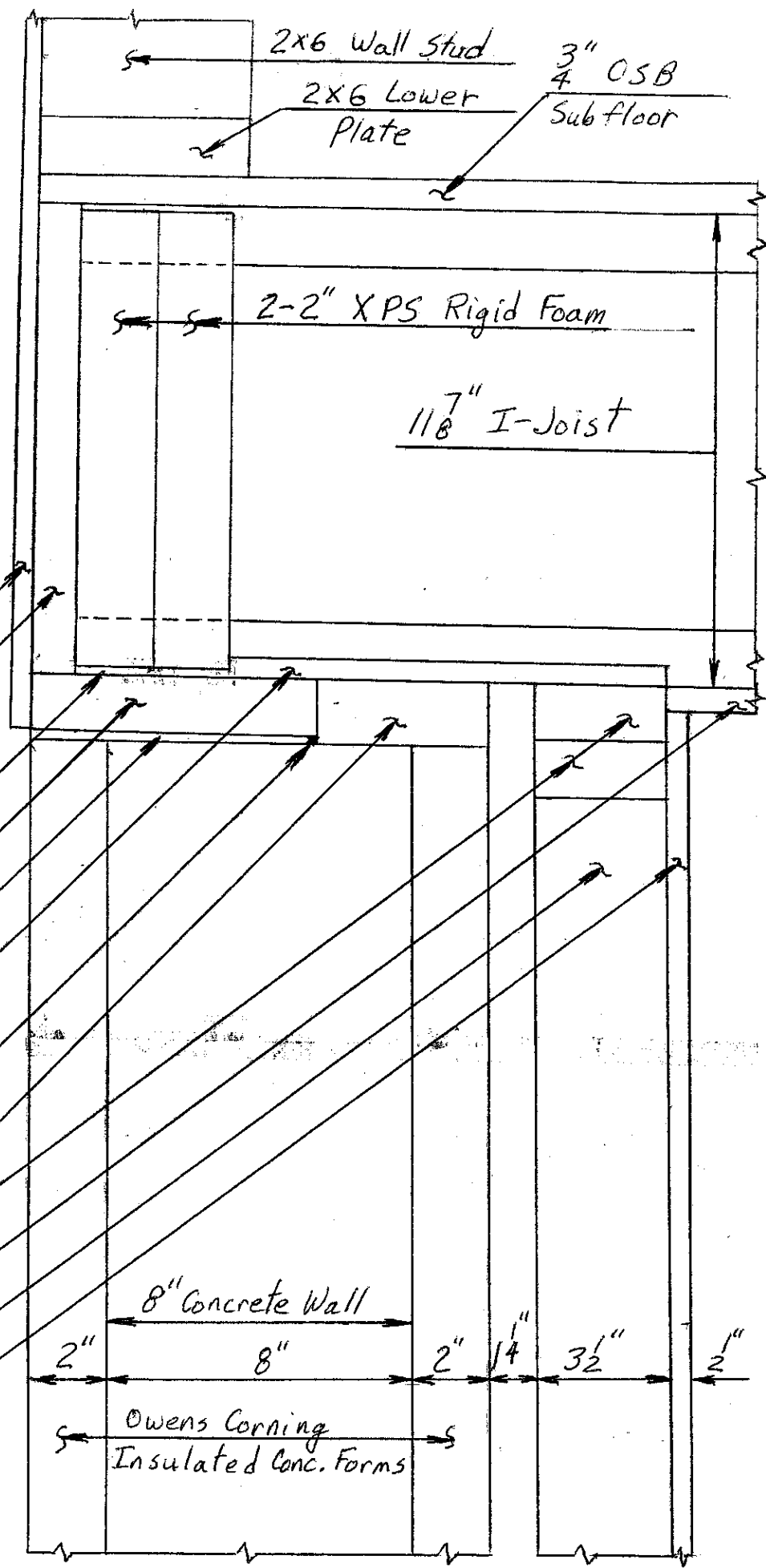
SECTION A-A
