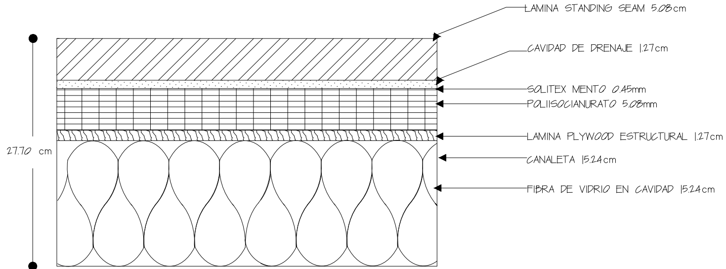
DETALLE COMUN DE TECHO
