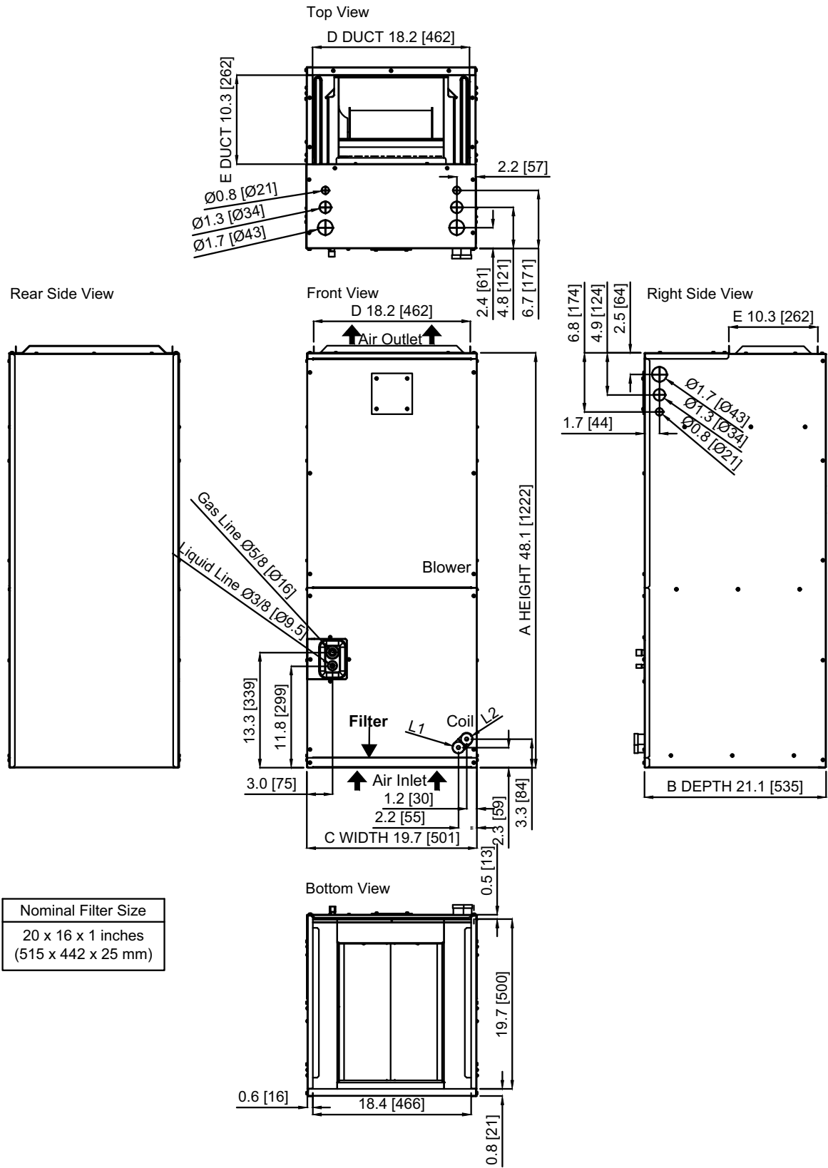
Fig. 3 — Dimensions
